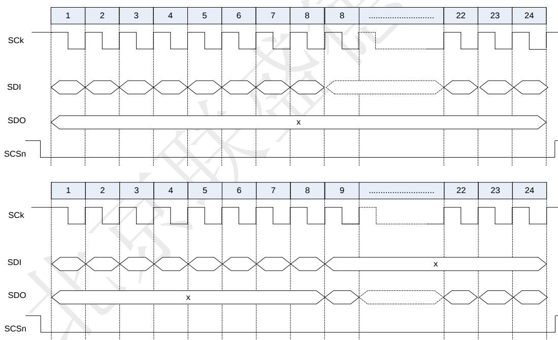
图 17 CPOL=1,CPHA=0
