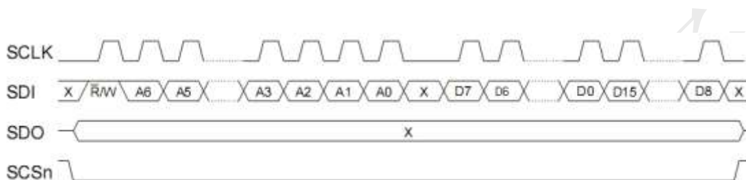
图 10 寄存器写操作(小端模式)
