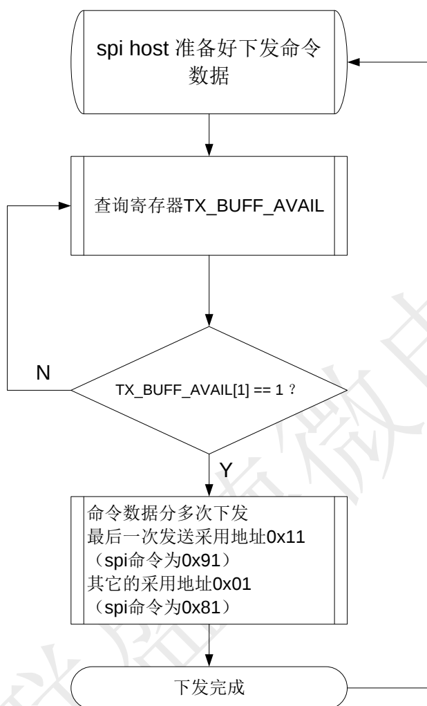
图 21 下行命令流程图
