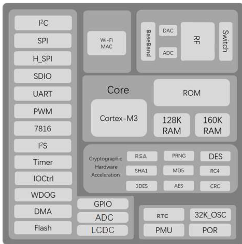
图 1 W601 芯片结构图
