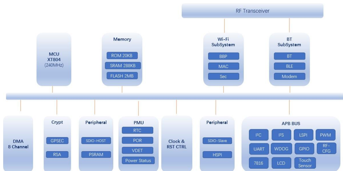
图 3-1 W801 芯片结构图
