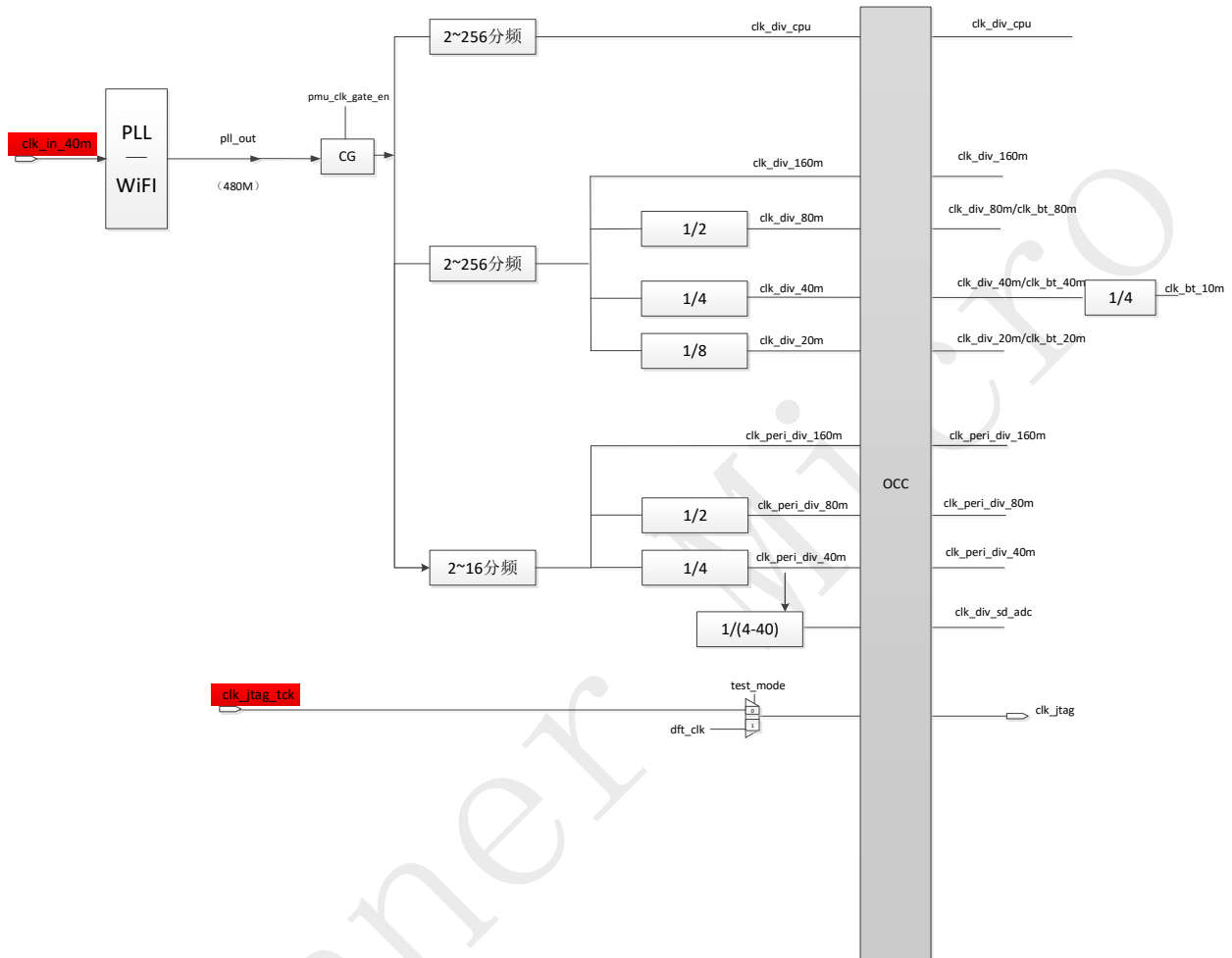
图 3 W801 时钟结构
