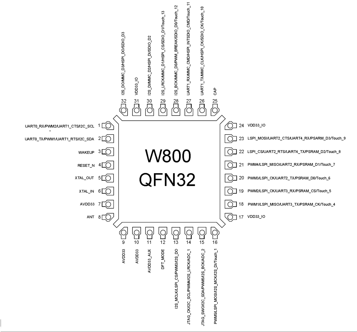
图 38 W801 芯片引脚分布
