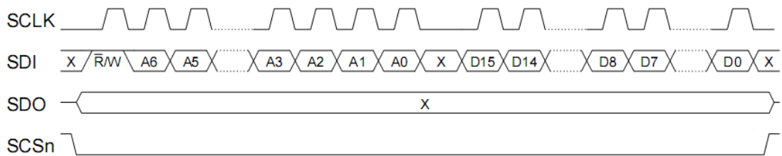
图 7 HSPI 寄存器写操作(大端模式)
