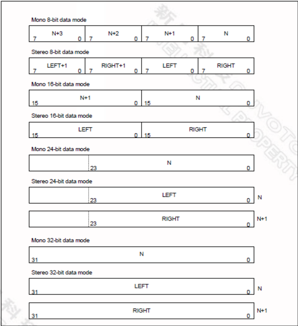
Fig 5. FIFO 存储结构
