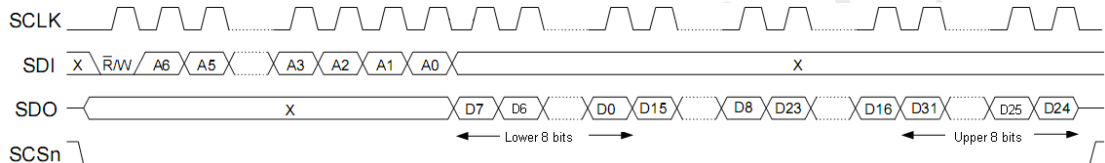
图 12 端口读操作(小端模式)
