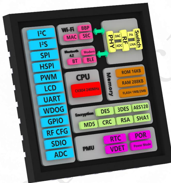
图 1 W801 芯片结构图
