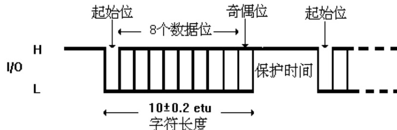
图 36 7816 数据传输
