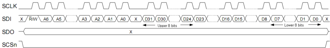
图 11 端口写操作(大端模式)
