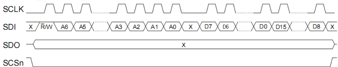
图 9 寄存器写操作(小端模式)
