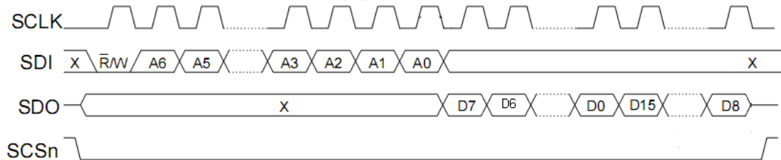
图 8 寄存器读操作(小端模式)
