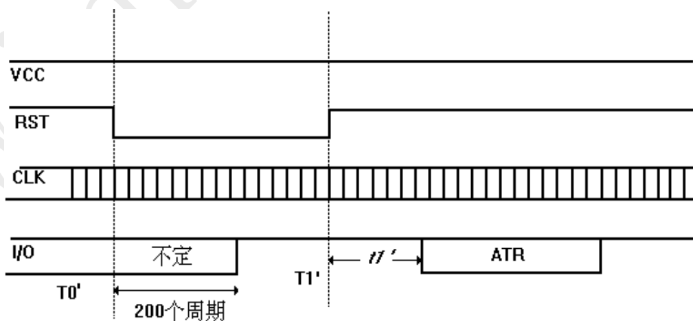
图 34 7816 热复位
