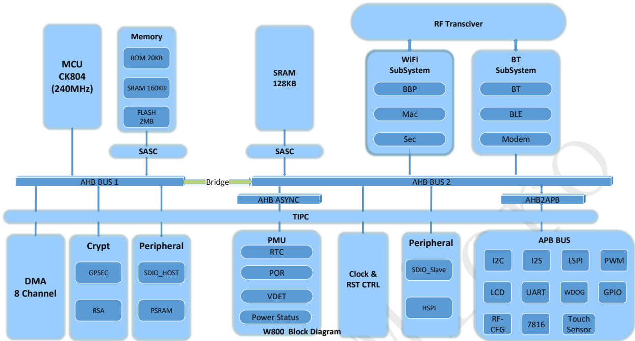
图 2 W801 总线结构图
