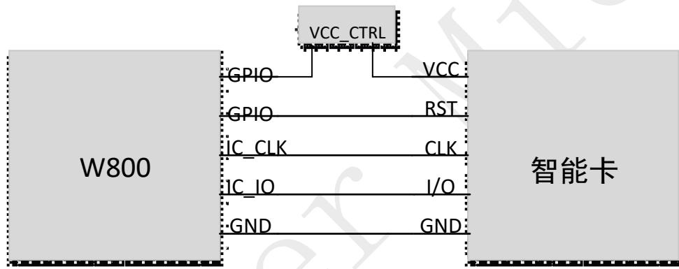
图 32 7816 连接示意图
