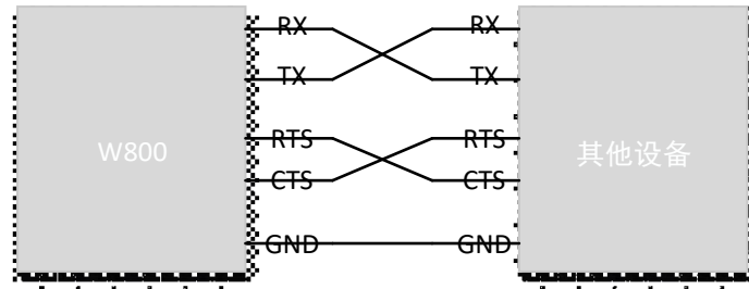
图 31 UART 硬件流控连接
