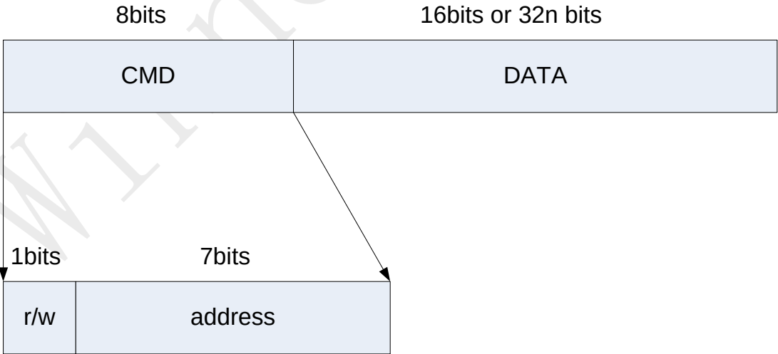
图 5 上位机 SPI 收发数据格式
