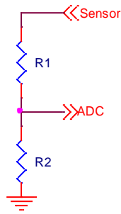
图 4-1 ADC 分压电路
